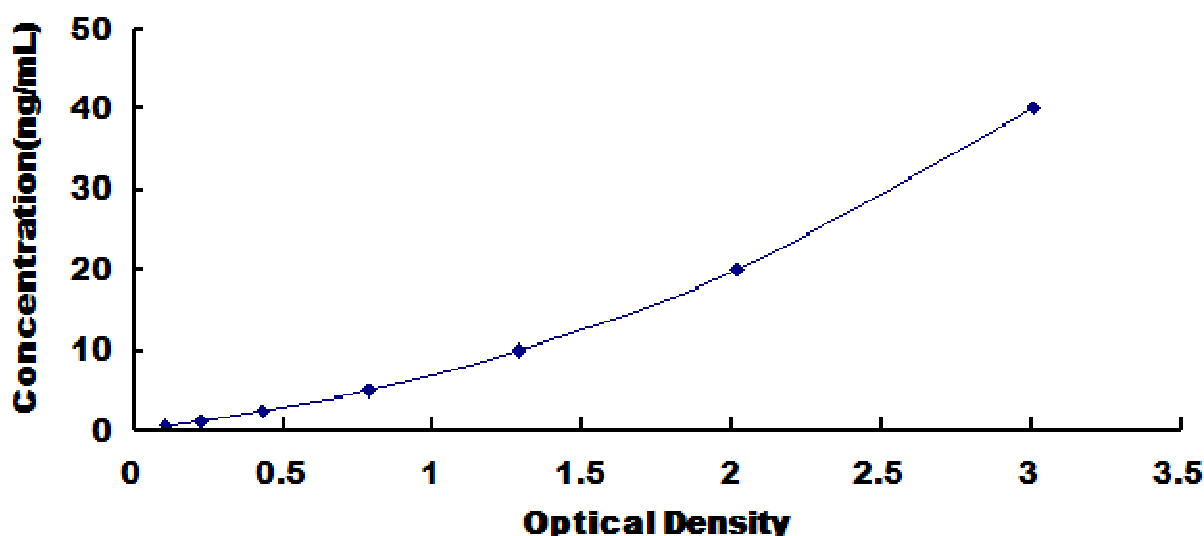
人干扰素 \alpha / \beta 受体 2(IFN \alpha / \beta R2) 检测试剂盒标准曲线
