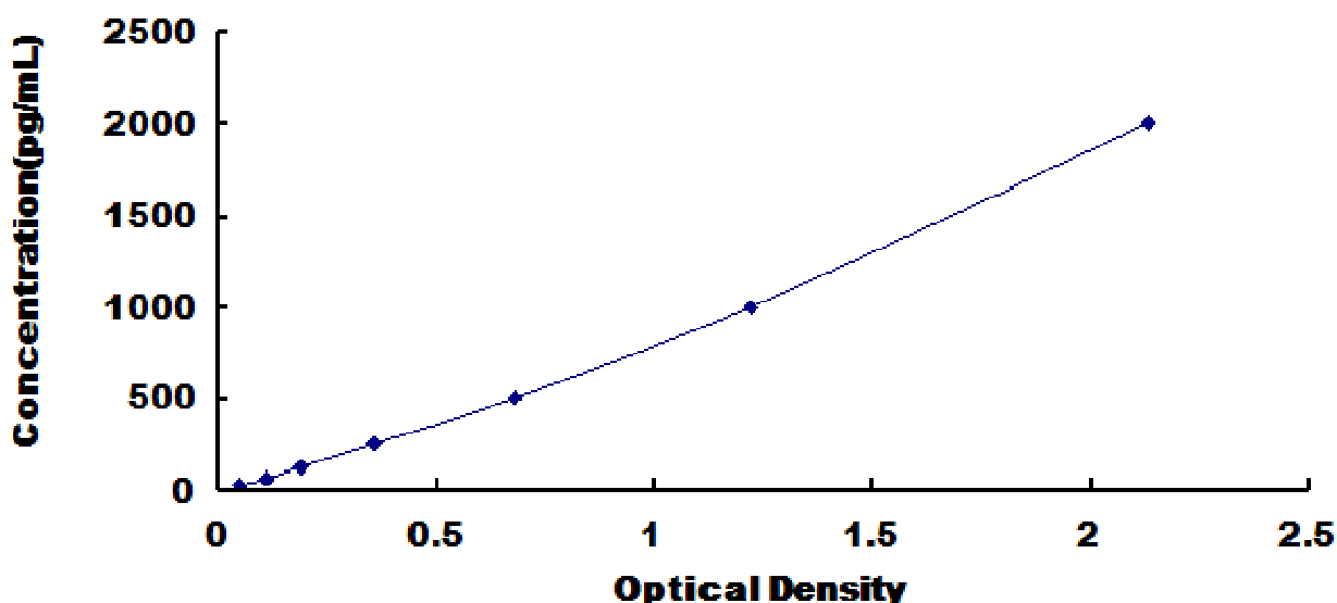
马干扰素 \beta (IFN \beta ) 检测试剂盒标准曲线
