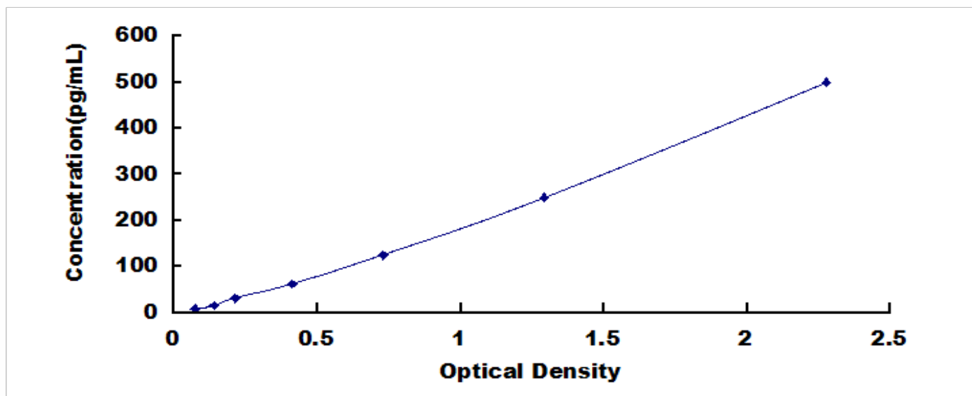
人干扰素 \beta (IFN \beta ) 检测试剂盒标准曲线
