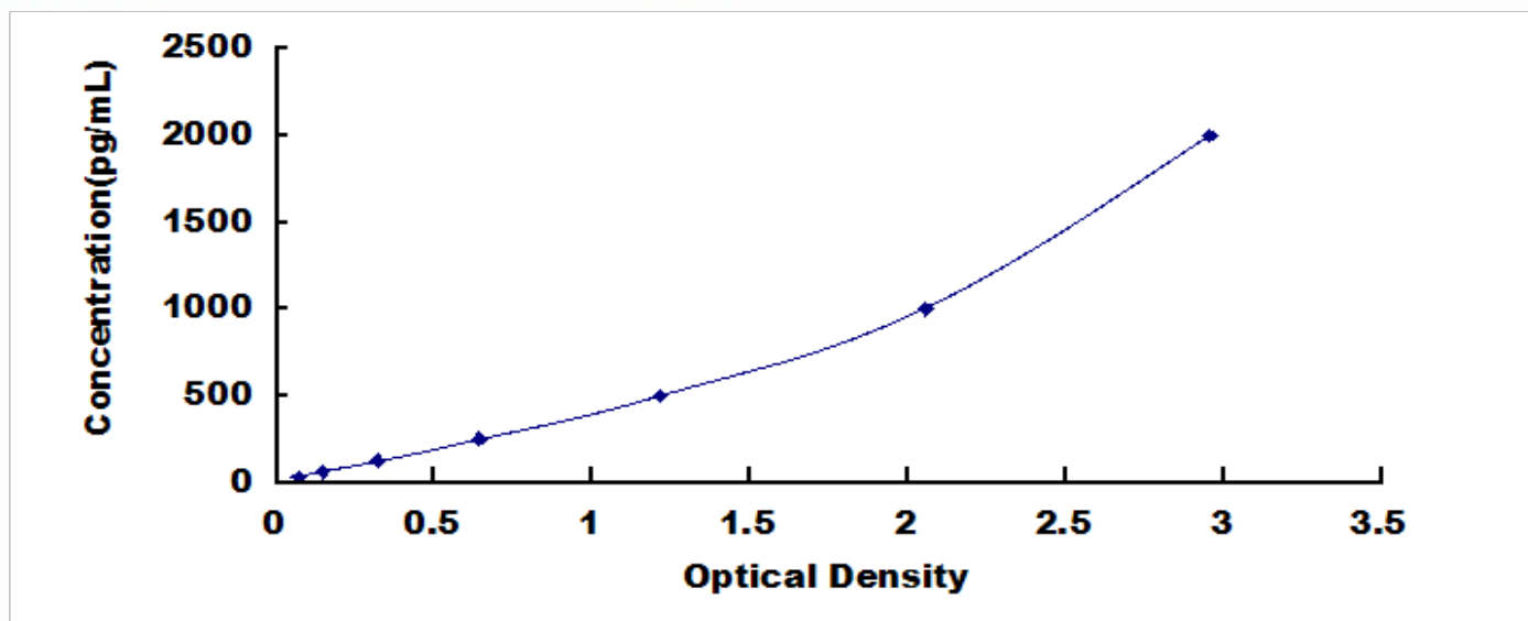
人 10kDa 干扰素 \gamma 诱导蛋白 (IP10) 检测试剂盒标准曲线
