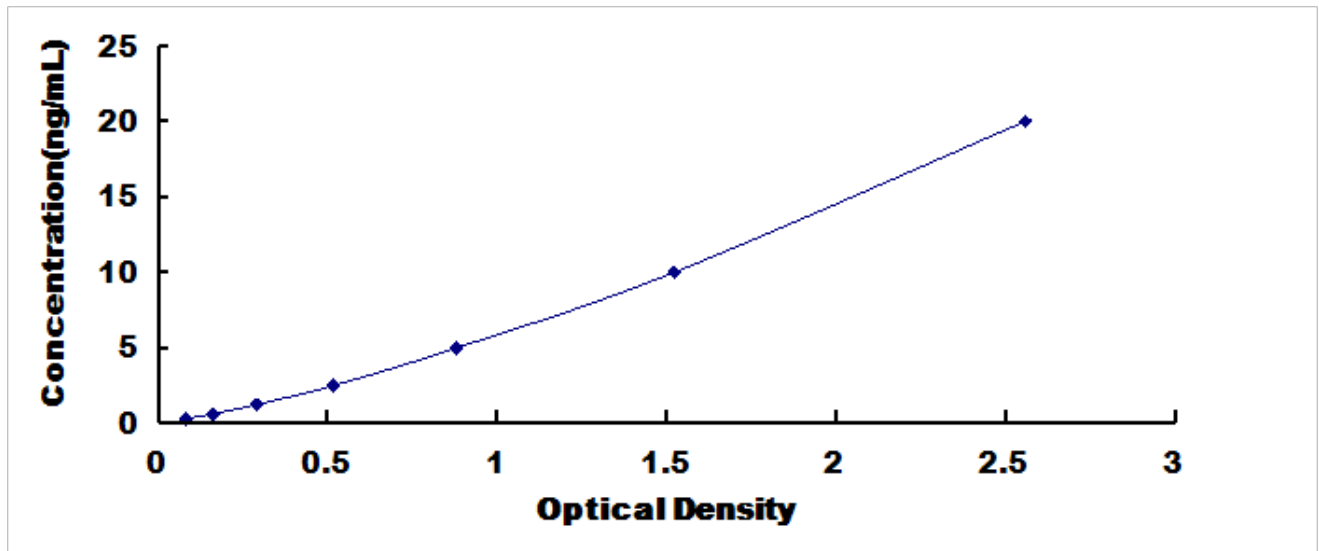
大鼠干扰素调节因子 4 (IRF4) 检测试剂盒标准曲线
