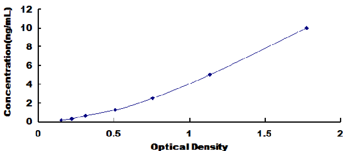
人干扰素调节因子 5 (IRF5) 检测试剂盒标准曲线
