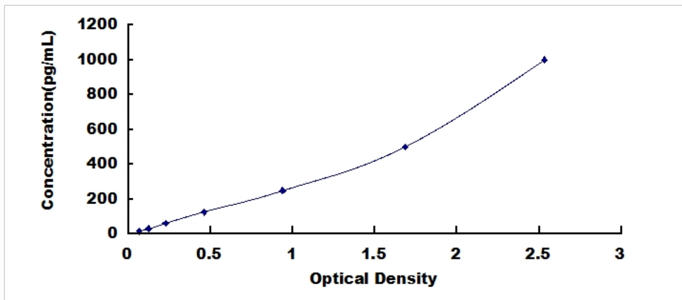
牛白介素 1 \beta (IL1 \beta ) 检测试剂盒标准曲线
