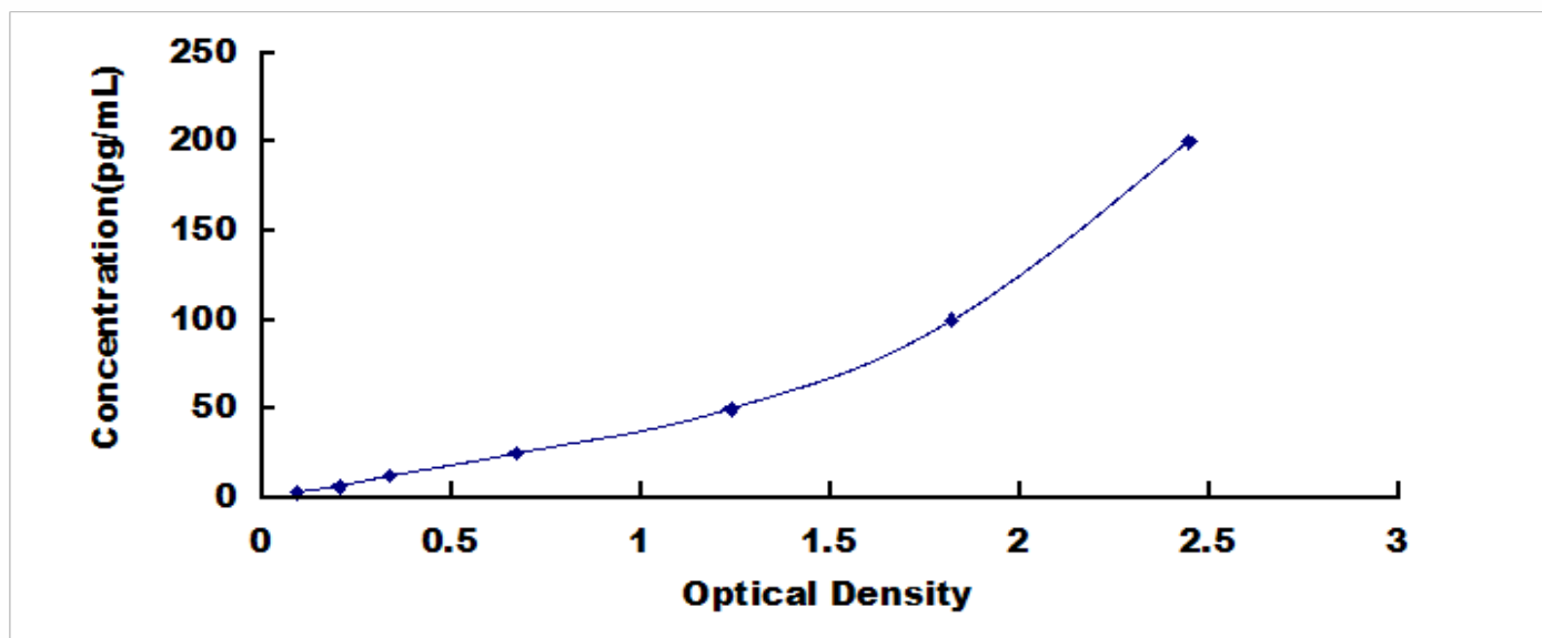
兔白介素 1 \beta (IL1 \beta )检测试剂盒标准曲线
