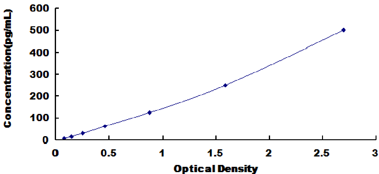
小鼠白介素 1 家族成员 9(IL1F9) 检测试剂盒标准曲线
