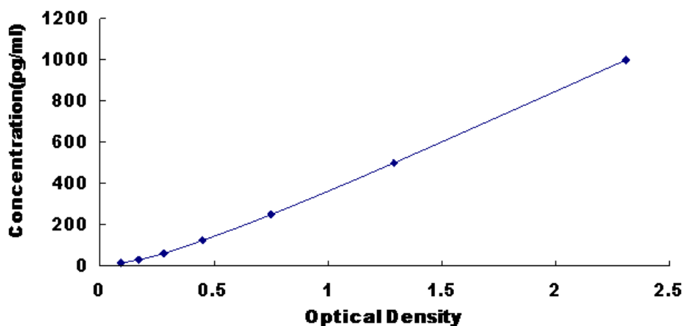
图 1: 大鼠白介素 11(IL11)试剂盒标准曲线
