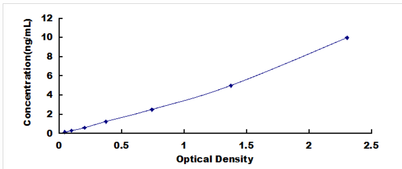
人白介素 12 受体 \beta 2 (IL2R \beta 2) 检测试剂盒标准曲线
