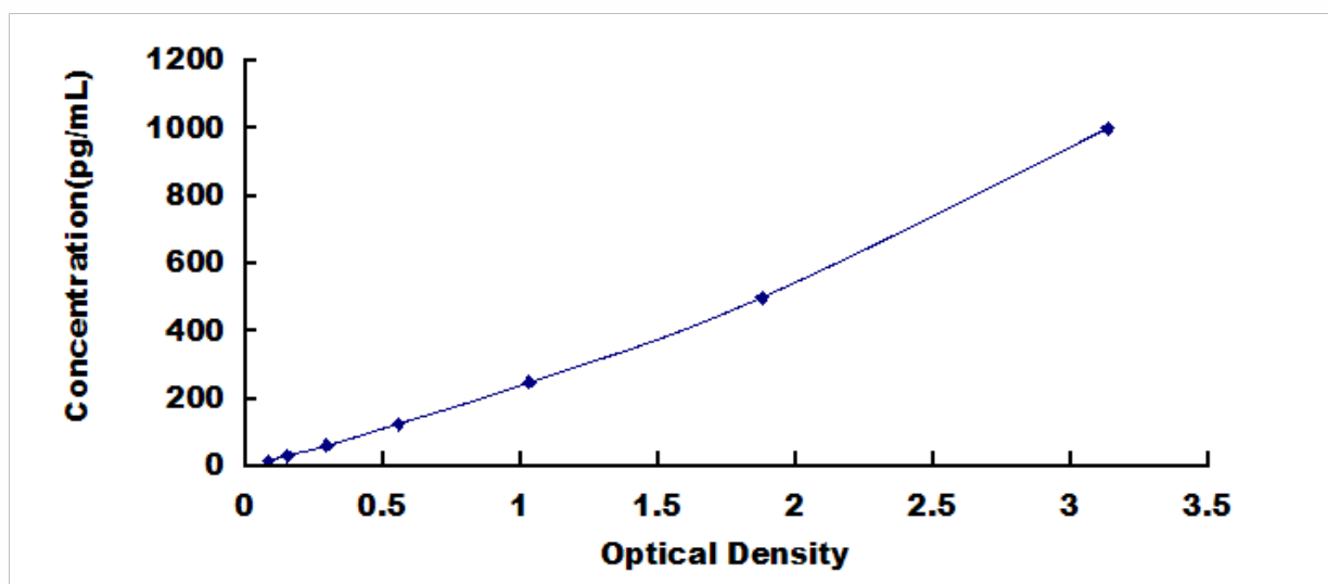
人白介素 16 (IL16) 检测试剂盒标准曲线
