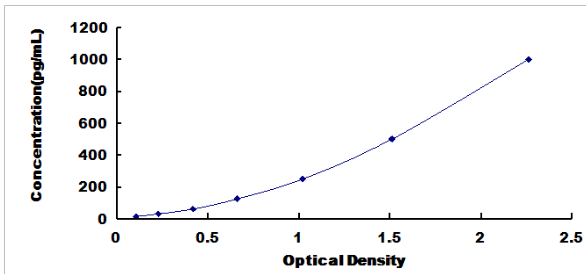
人白介素 17 (IL17) 检测试剂盒标准曲线
