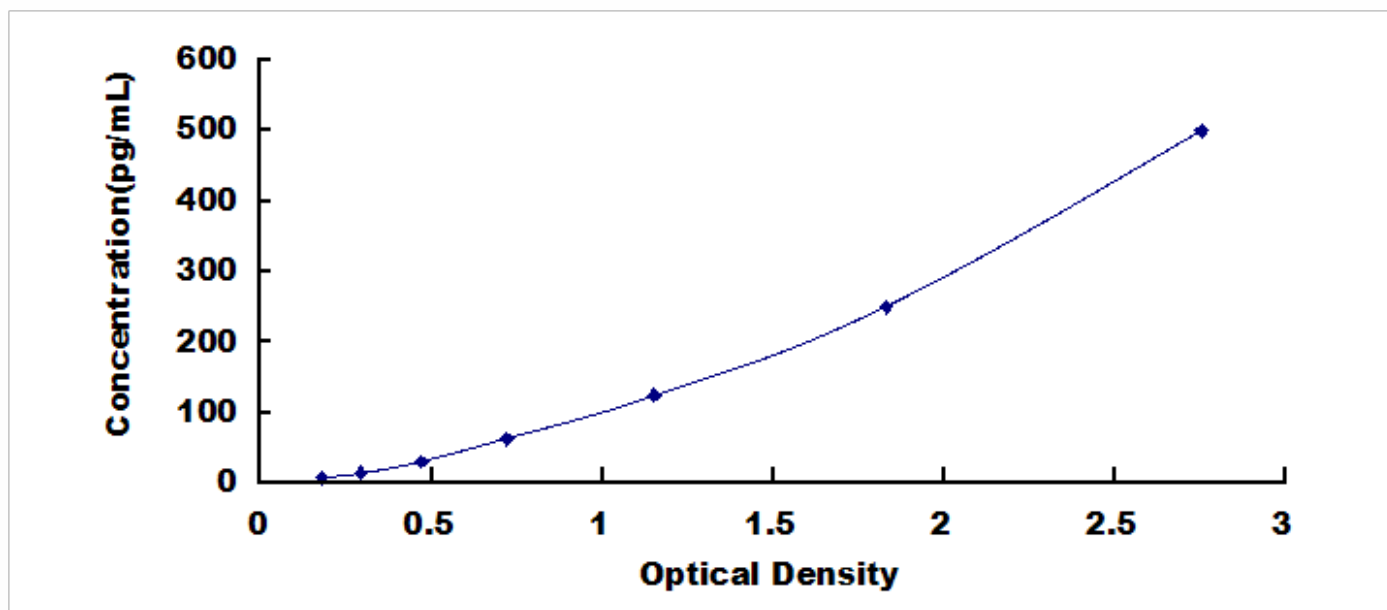
人白介素 17D (IL17D) 检测试剂盒标准曲线
