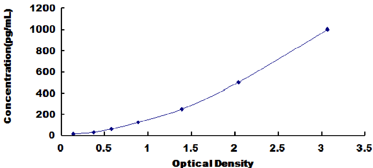
猪白介素 18 (IL18) 检测试剂盒标准曲线
