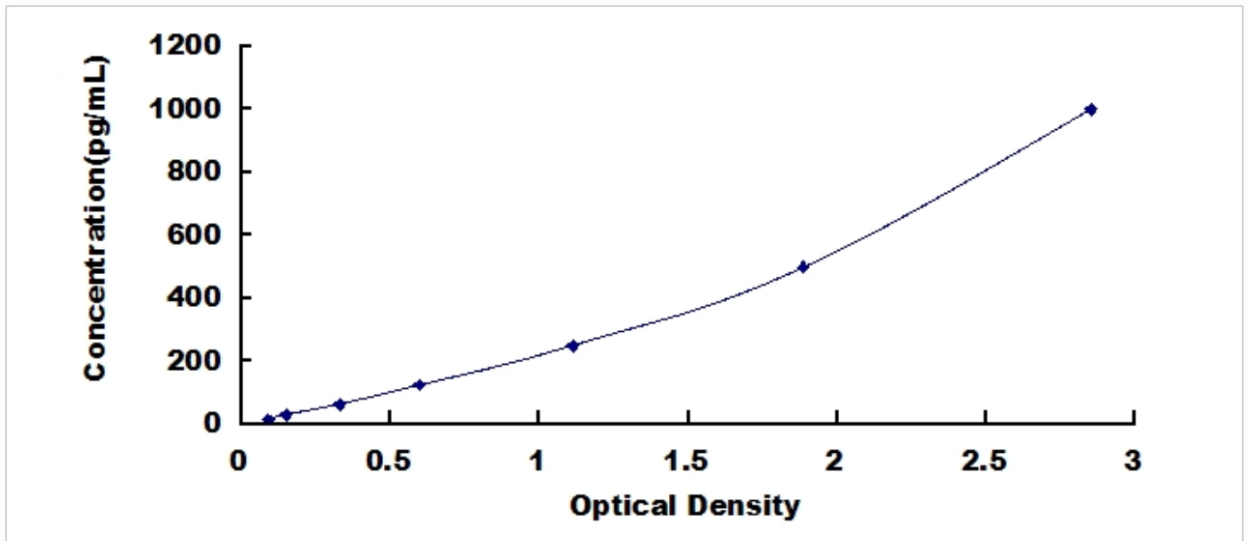
人白介素 18(IL18)检测试剂盒标准曲线
