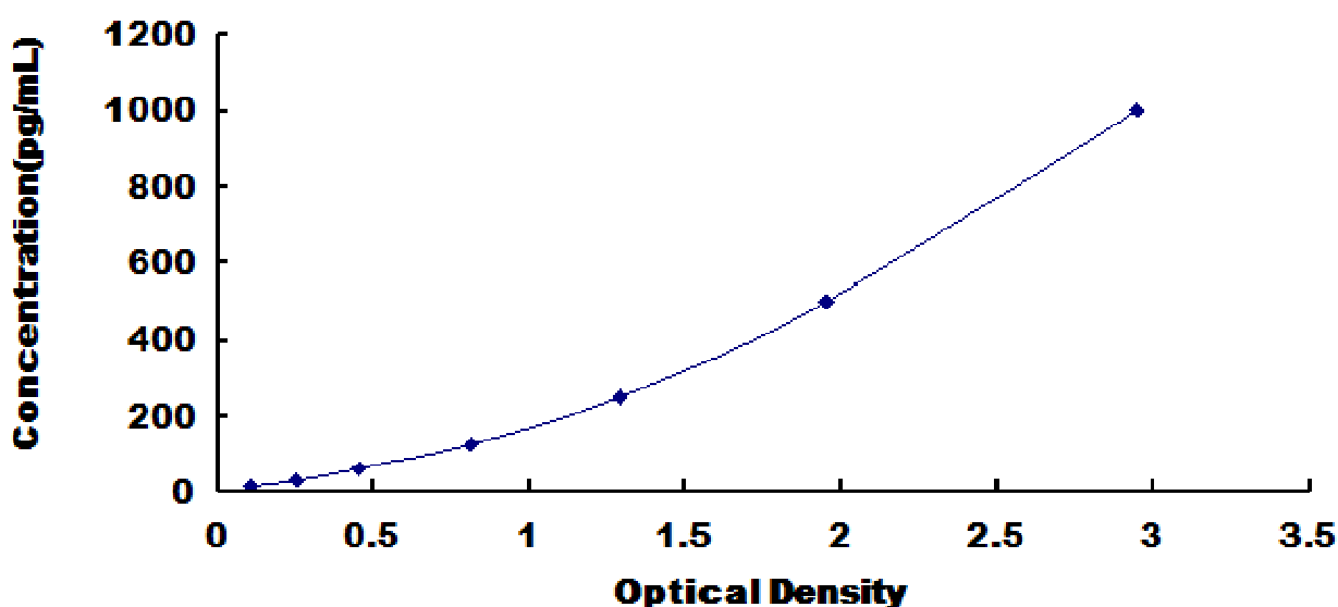
鸡白介素 2(IL2)检测试剂盒标准曲线
