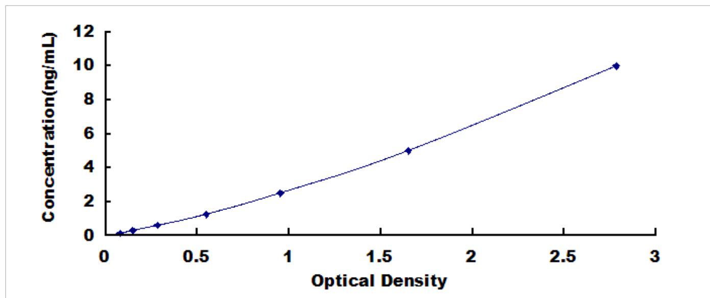
人白介素 2 受体 \gamma (IL2R \gamma ) 检测试剂盒标准曲线
