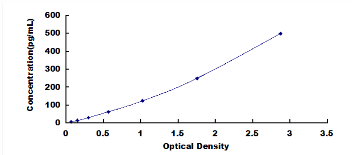
人白介素 22 (IL22) 检测试剂盒标准曲线
