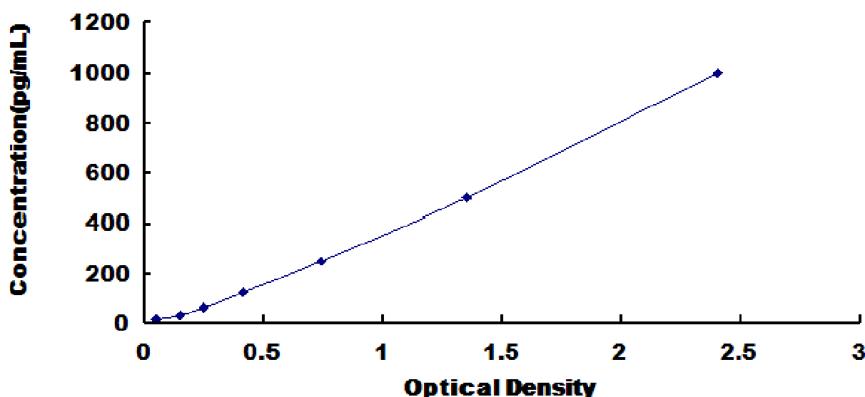
小鼠白介素 25 (IL25) 检测试剂盒标准曲线
