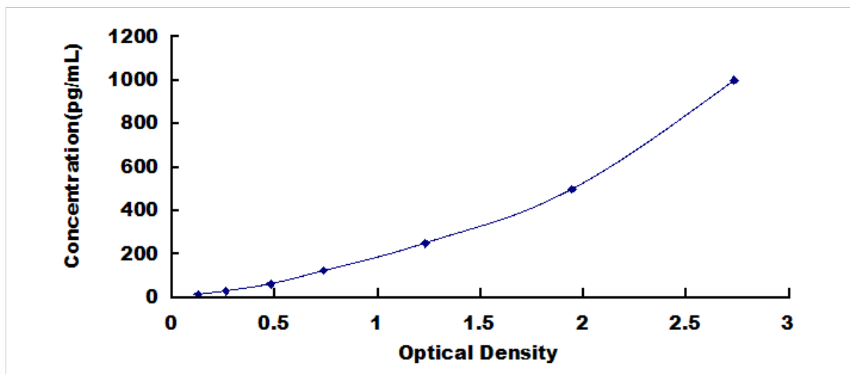
人白介素 26 (IL26) 检测试剂盒标准曲线
