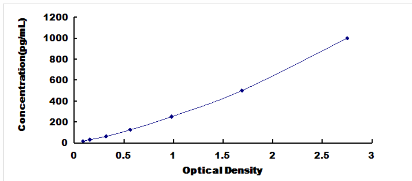
人白介素 27(IL27)检测试剂盒标准曲线
