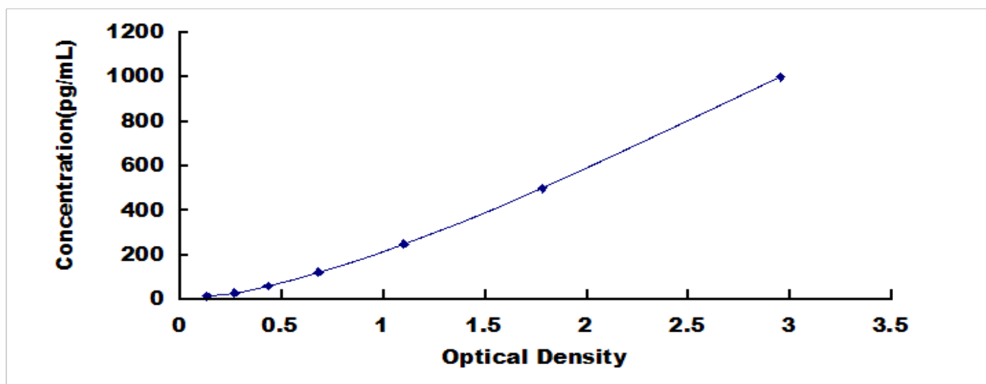
人白介素 34(IL34)检测试剂盒标准曲线
