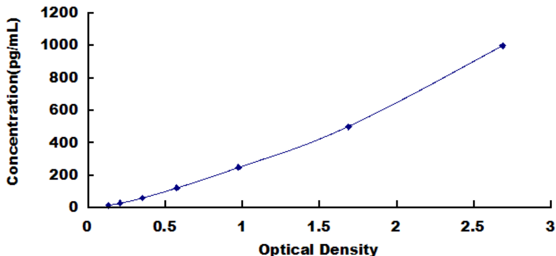
人白介素 4(IL4) 检测试剂盒标准曲线
