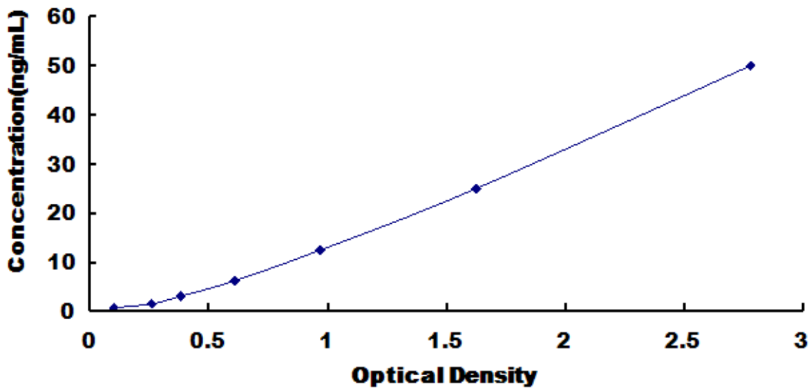
大鼠白介素 6 受体(IL6R)试剂盒标准曲线
