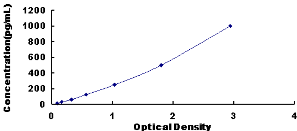
图 1: 犬的白介素 8(IL8)试剂盒标准曲线
