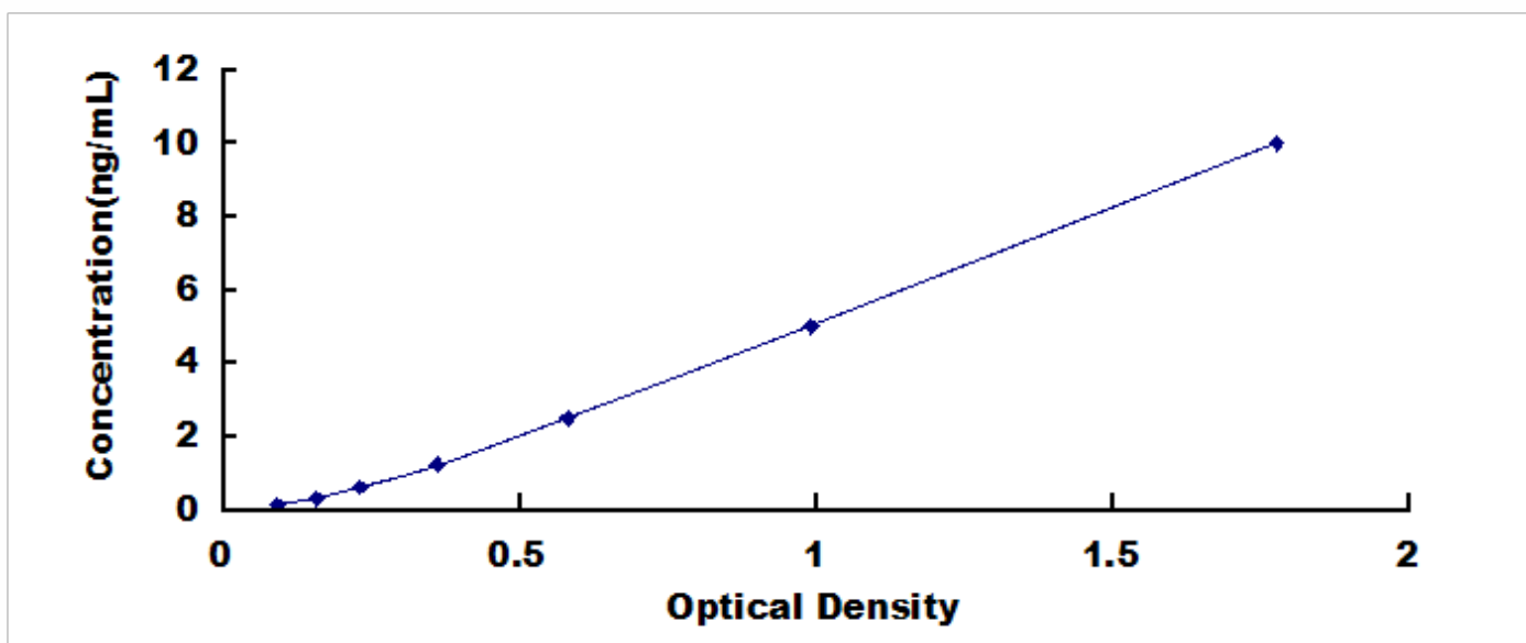
人白介素 8 受体 \alpha (IL8R \alpha ) 检测试剂盒标准曲线
