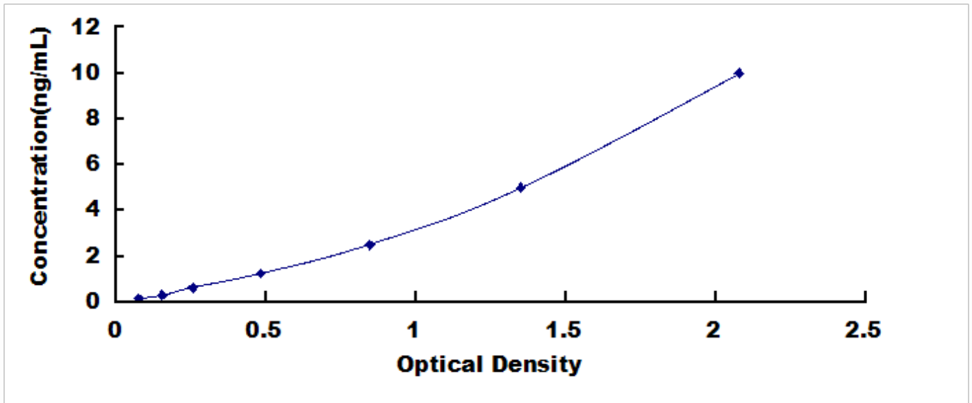
人白介素 8 受体 \alpha (IL8R \alpha ) 检测试剂盒标准曲线
