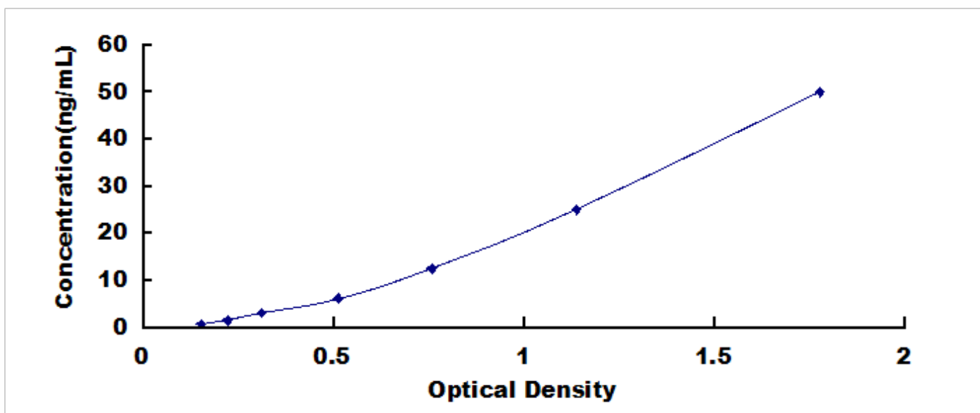
人白介素 8 受体 \beta (IL8R \beta ) 检测试剂盒标准曲线
