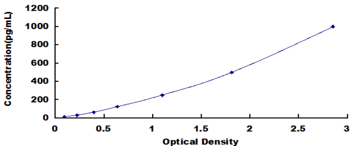
人白介素 9 (IL9) 检测试剂盒标准曲线
