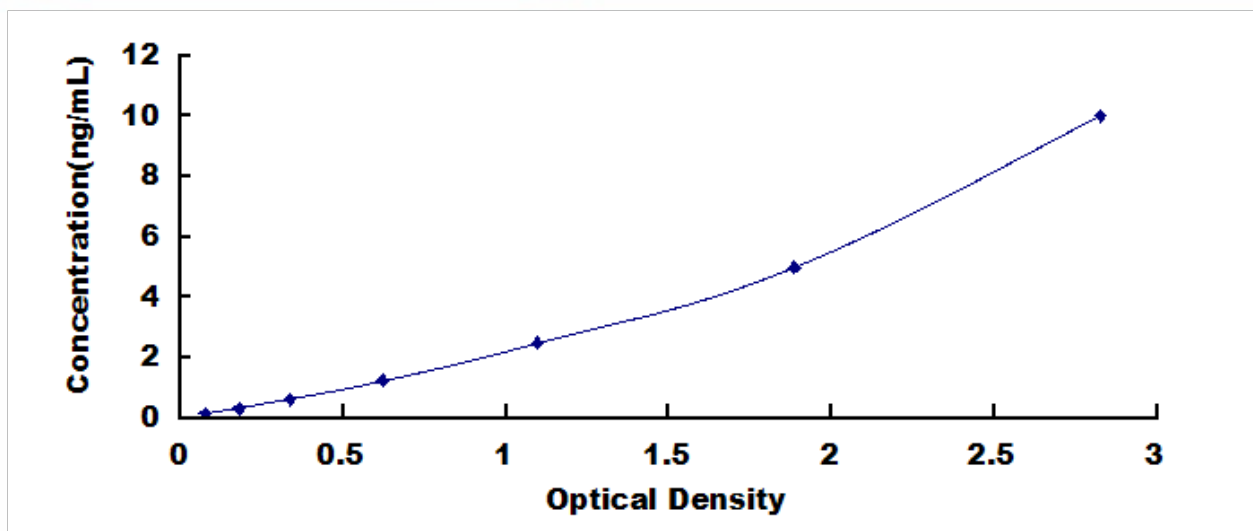
人异柠檬酸脱氢酶 2 (IDH2) 检测试剂盒标准曲线
