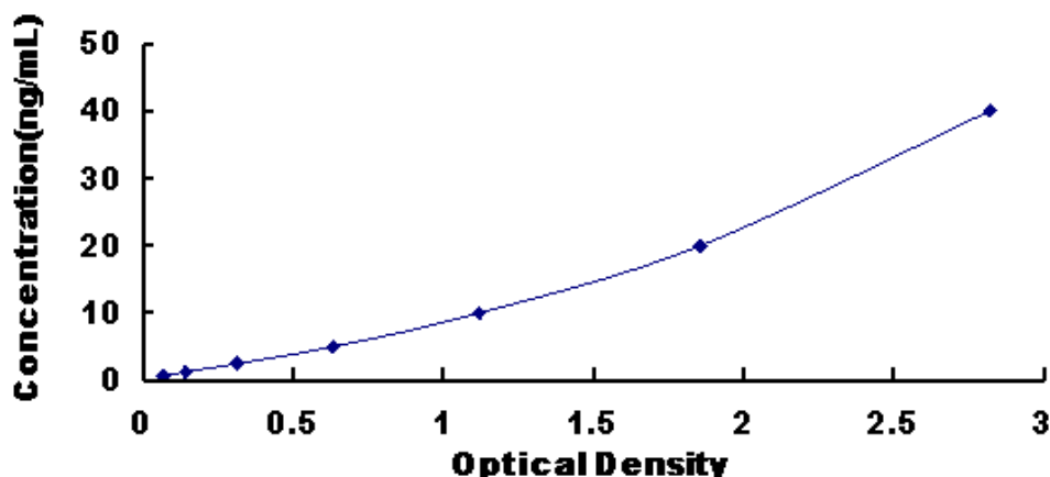
图 1：人的激肽释放酶 10(KLK10)试剂盒标准曲线
