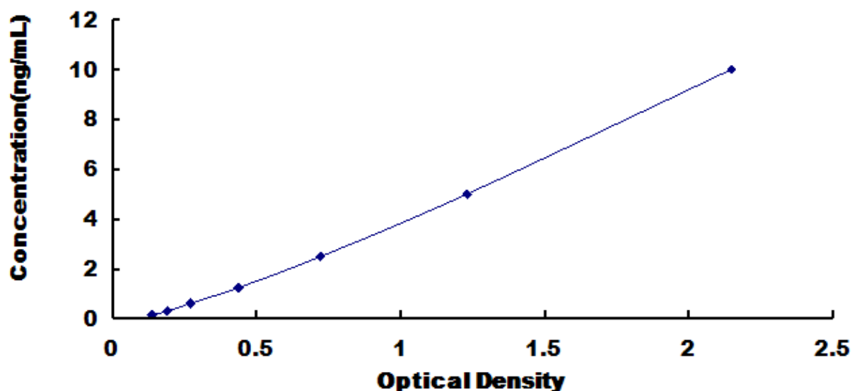
小鼠激肽释放酶 3 (KLK3) 试剂盒标准曲线
