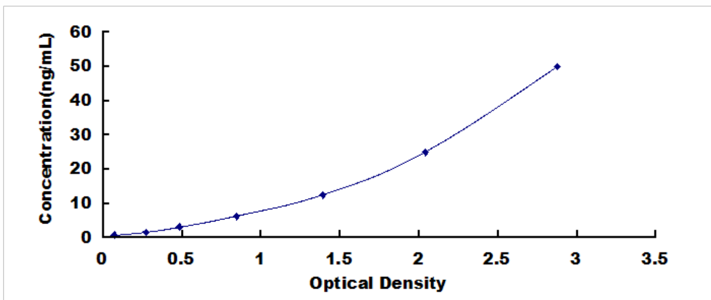
人 Ki-67 蛋白 (Ki67P) 检测试剂盒标准曲线
