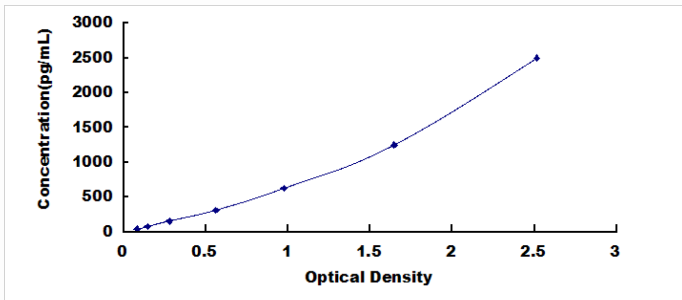
小鼠肾损伤分子 1 (Kim1) 检测试剂盒标准曲线
