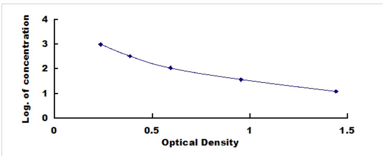
小鼠吻素 1 (KISS1) 检测试剂盒标准曲线
