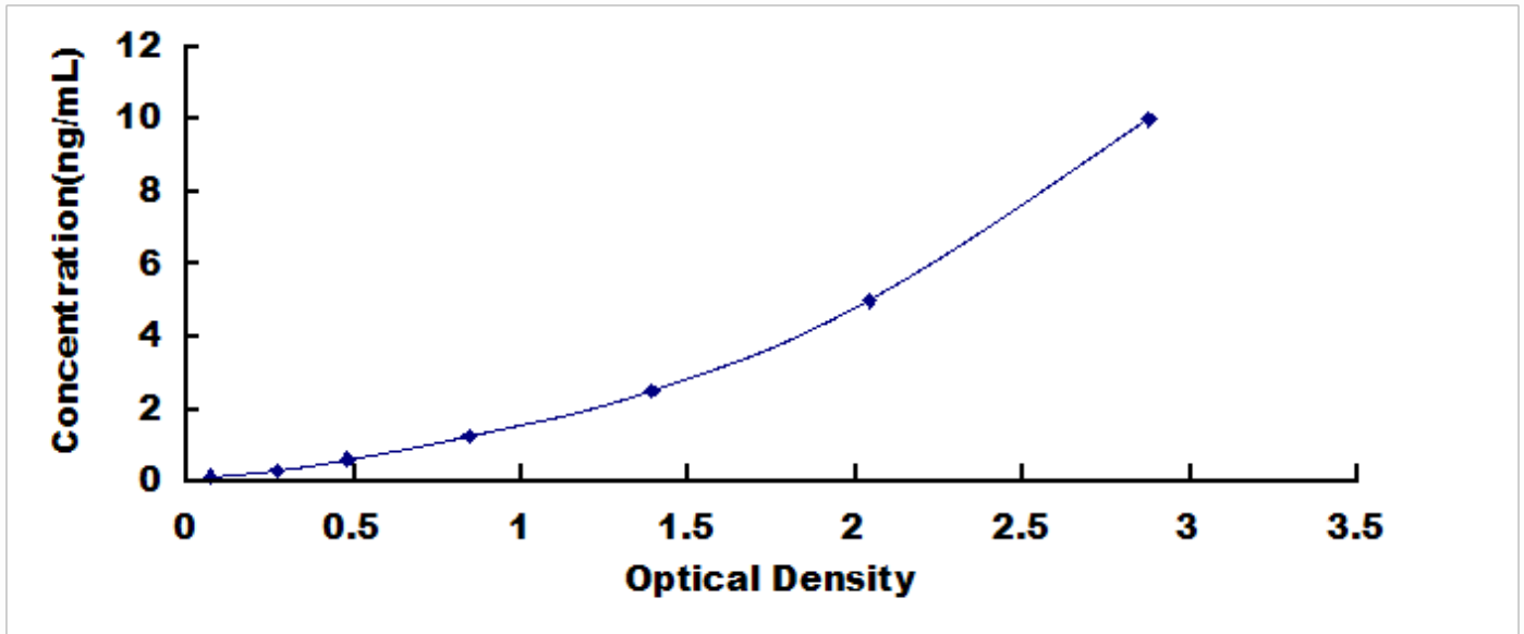
人 Kruppel 样因子 2 (KLF2) 检测试剂盒标准曲线
