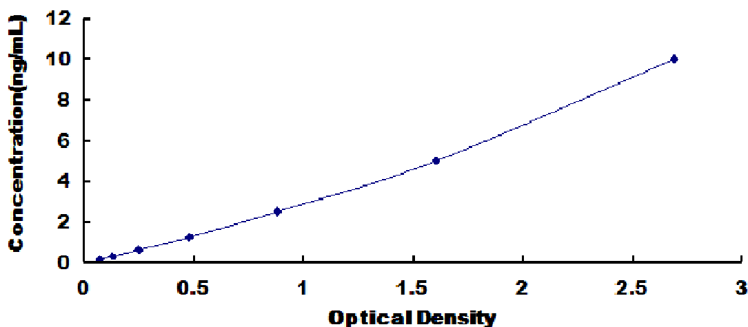
人犬尿酸酶(KYNU)检测试剂盒标准曲线
