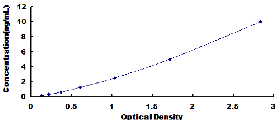
小鼠乳酸脱氢酶(LDH)检测试剂盒标准曲线
