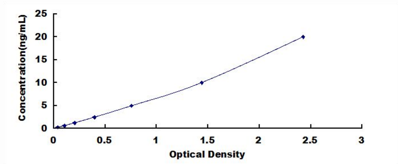
大鼠乳酸脱氢酶 B (LDHB) 检测试剂盒标准曲线
