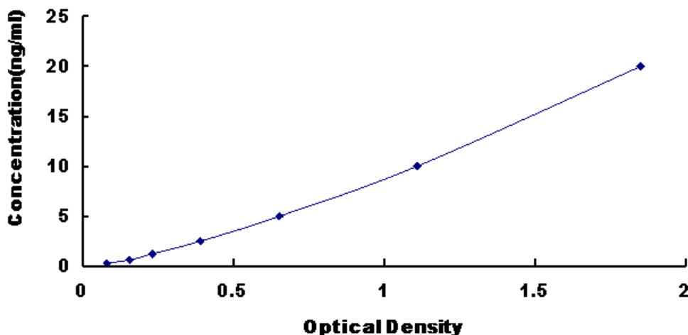
图 1: 大鼠乳铁传递蛋白(LTF)试剂盒标准曲线
