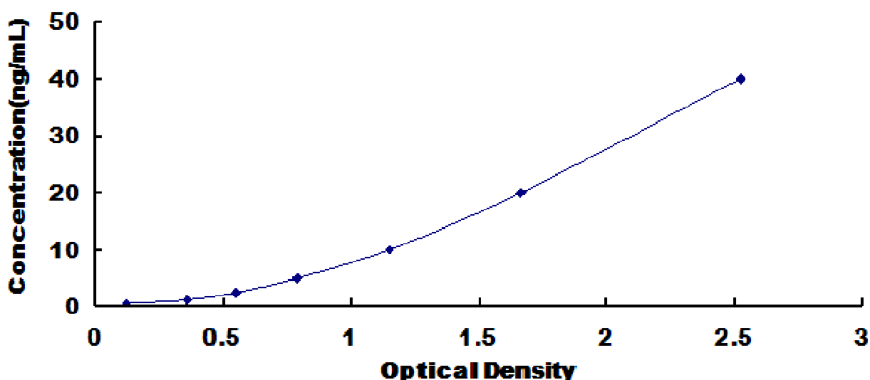
人层黏连蛋白 \alpha 4 (LAM \alpha 4) 检测试剂盒标准曲线
