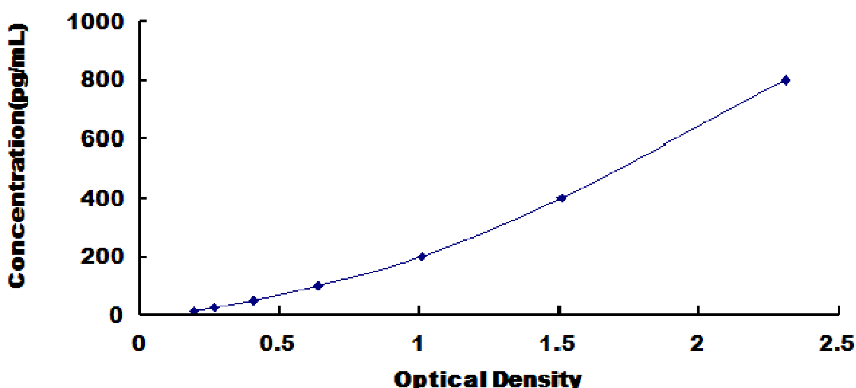
小鼠凝集素样氧化低密度脂蛋白受体 1 (LOX1) 检测试剂盒标准曲线
