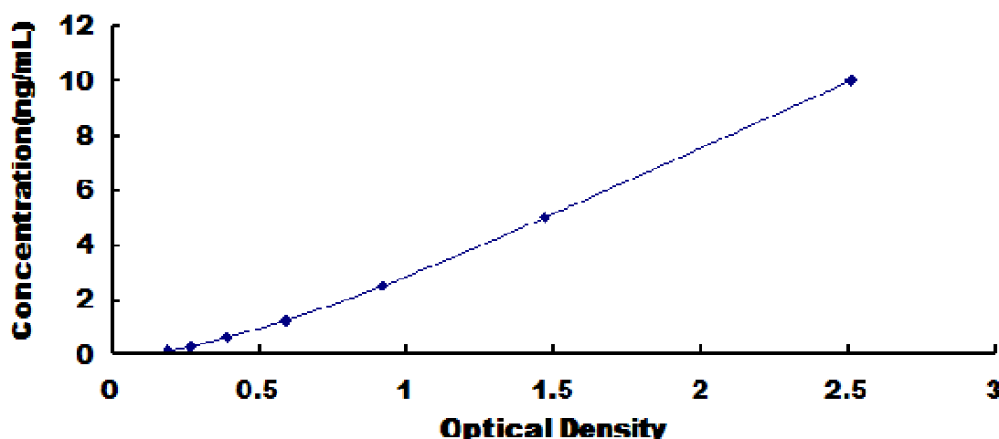
人 Lemur 酪氨酸激酶 3(LMTK3) 检测试剂盒标准曲线
