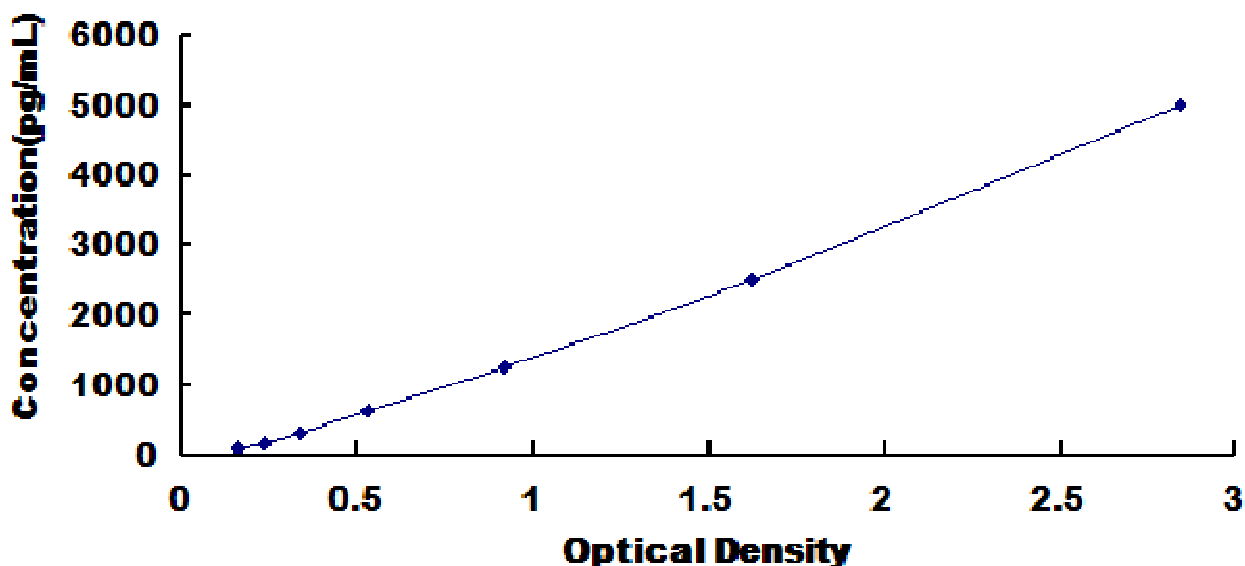
人白血病抑制因子(LIF)试剂盒标准曲线
