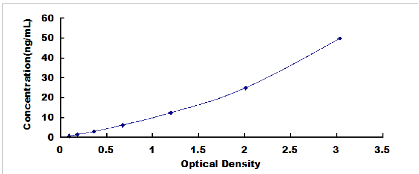
人白细胞衍生趋化因子 2 (LECT2) 检测试剂盒标准曲线
