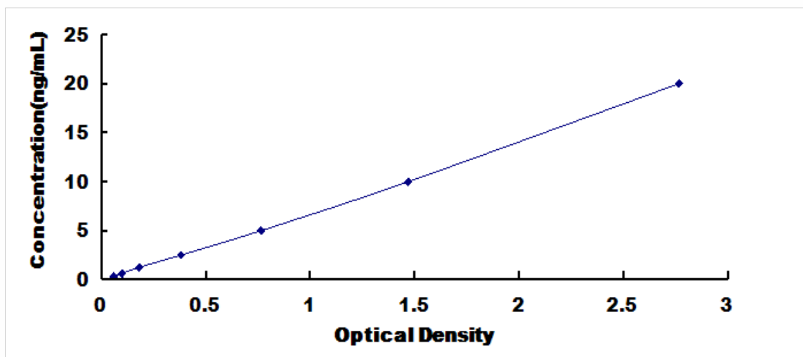
人白细胞免疫球蛋白样受体亚家族 A 成员 3 (LILRA3) 检测试剂盒标准曲线
