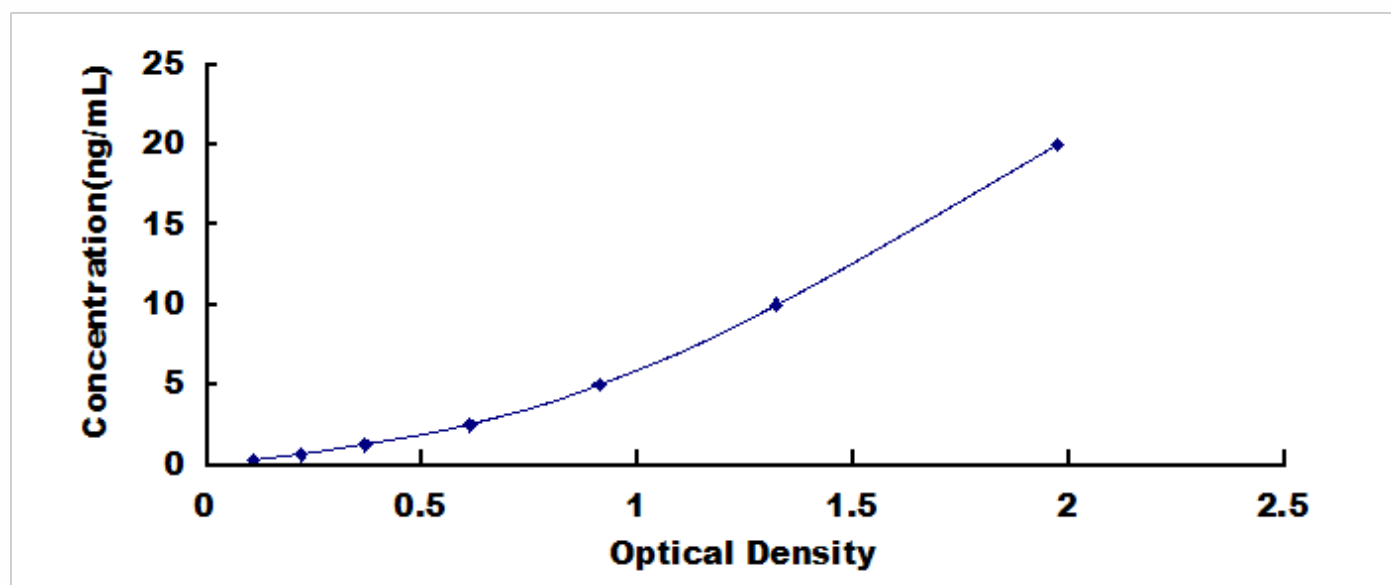
大鼠脂蛋白脂酶(LIPD)检测试剂盒标准曲线
