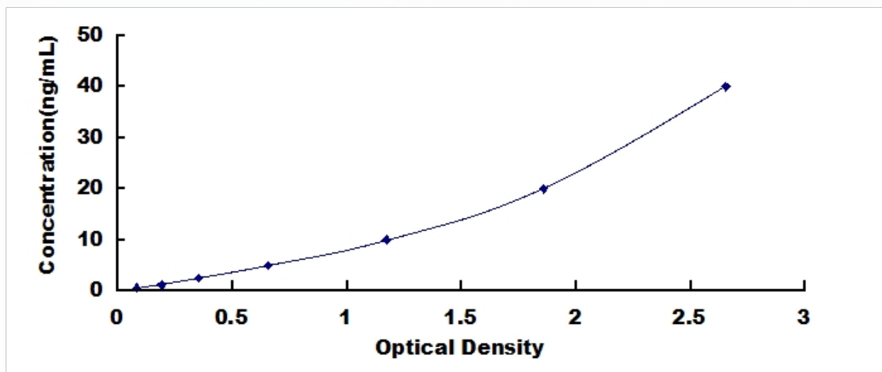
牛脂多糖结合蛋白 (LBP) 检测试剂盒标准曲线
