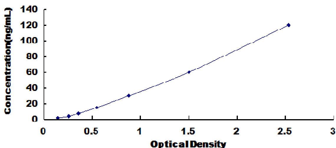
大鼠脂多糖结合蛋白(LBP)试剂盒标准曲线
